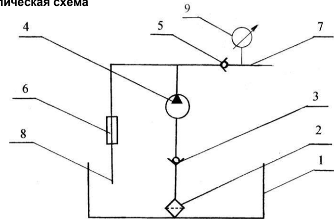
Рис. 1 Гидравлическая схема
